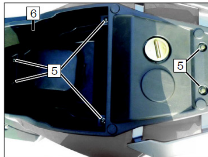
4. Retirar os parafusos (5) e a caixa de arrumos
