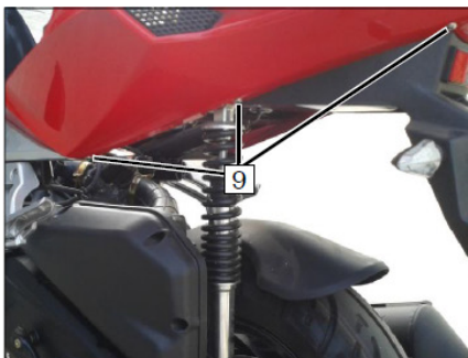
7. Retirar os parafusos (9) central
